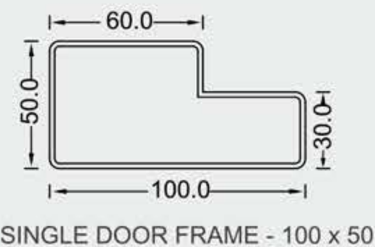
SINGLE DOOR FRAME - 100 x 50
